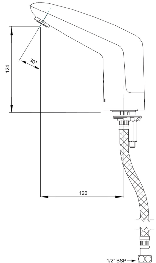
Presto Volta Sensor Tap - Mains
